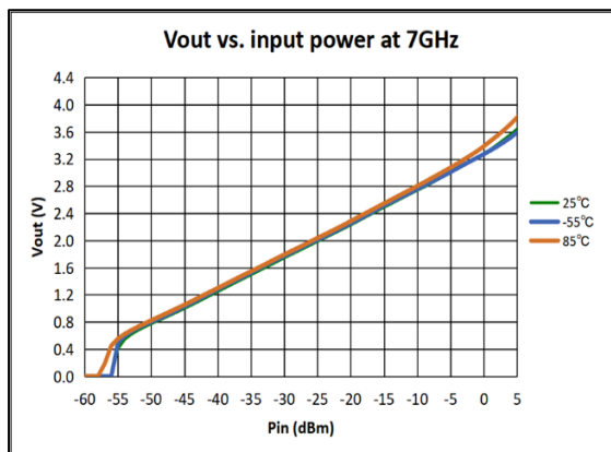
图 19 7000MHz 全温检波曲线
