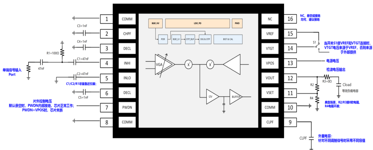
EMD211 单端典型连接框图
