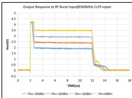
图 25 900MHz 输出瞬态响应，CLPF=Open
