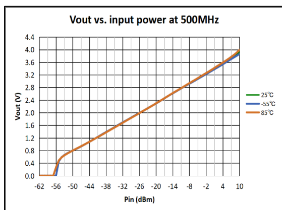
图 5 500MHz 全温检波曲线
