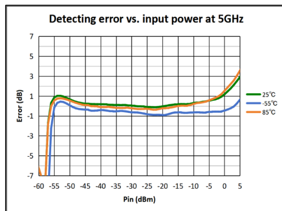
图 18 5000MHz 全温检波对数误差
