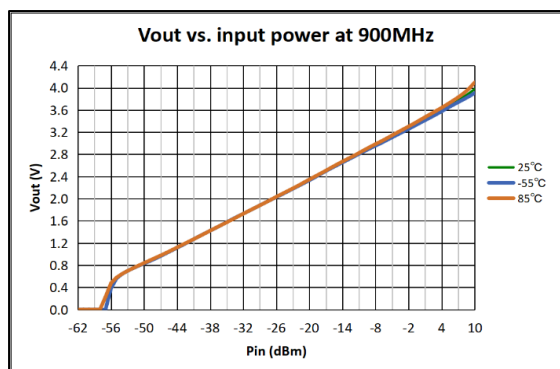
图 7 900MHz 全温检波曲线
