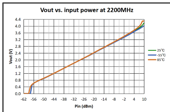
图 11 2200MHz 全温检波曲线
