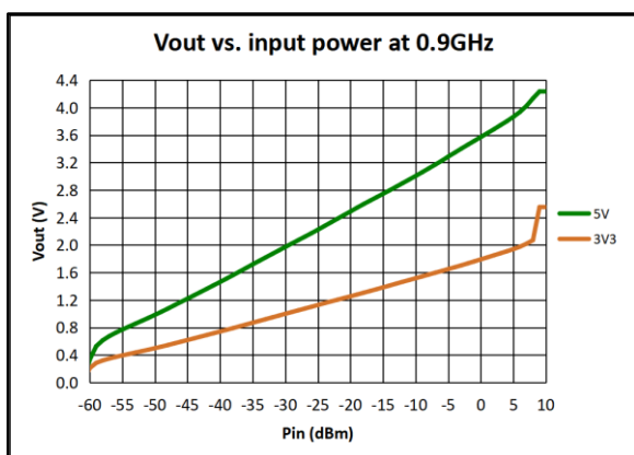
图 29 900MHz 检波曲线,VPOS=5V vs. 3V3
