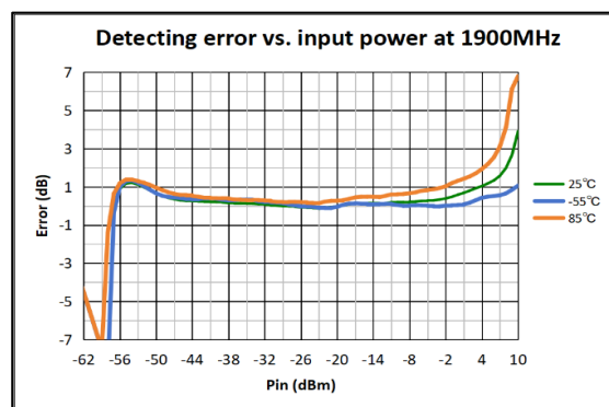
图 10 1900MHz 全温检波对数误差
