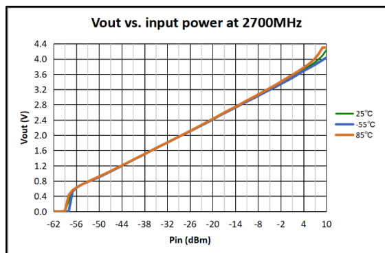
图 13 2700MHz 全温检波曲线
