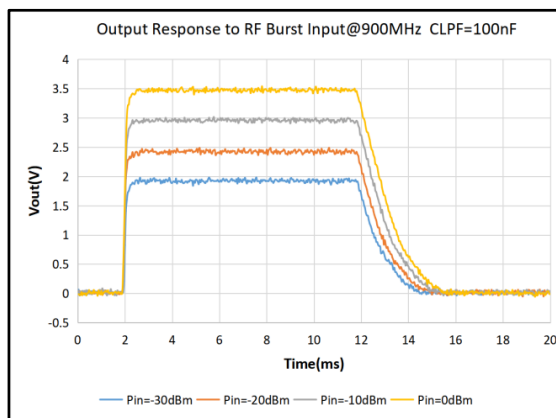
图 26 900MHz 输出瞬态响应，CLPF=0.1uF
