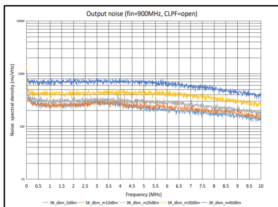
图 27 900MHz 输出噪声, CLPF=Open
