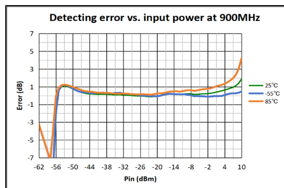
图 8 900MHz 全温检波对数误差
