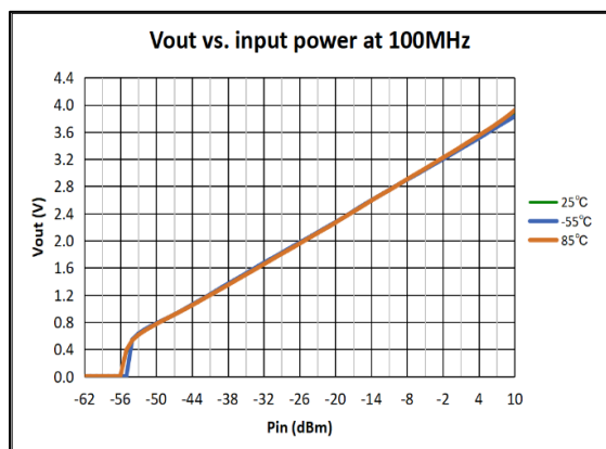
图 3 100MHz 全温检波曲线
