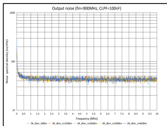
图 28 900MHz 输出噪声, CLPF=0.1uF
