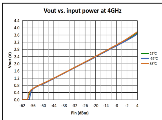
图 15 4000MHz 全温检波曲线
