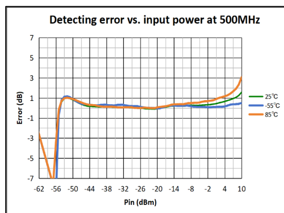
图 6 500MHz 全温检波对数误差
