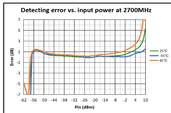
图 14 2700MHz 全温检波对数误差
