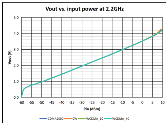
图 23 2200MHz 调制信号检波曲线
