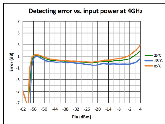
图 16 4000MHz 全温检波对数误差
