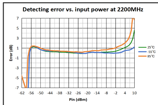
图 12 2200MHz 全温检波对数误差
