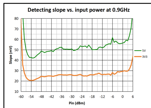
图 30 900MHz 检波曲线斜率,VPOS=5V vs. 3V3
