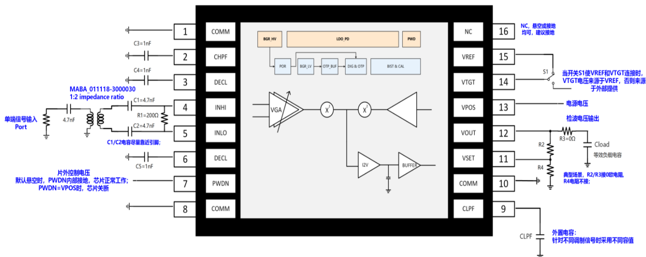
EMD211 差分典型连接框图
