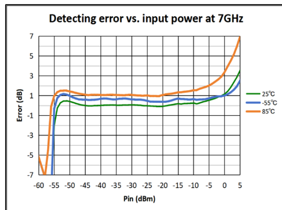
图 20 7000MHz 全温检波对数误差
