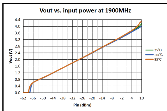
图 9 1900MHz 全温检波曲线
