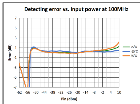
图 4 100MHz 全温检波对数误差
