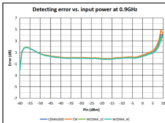
图 22 900MHz 调制信号检波对数误差
