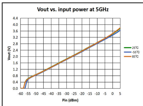
图 17 5000MHz 全温检波曲线
