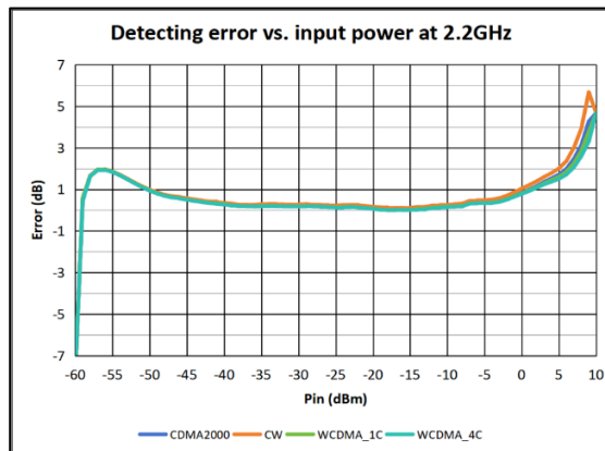
图 24 2200MHz 调制信号检波对数误差
