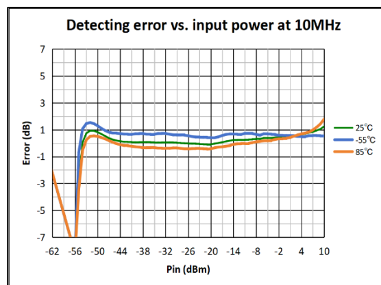
图 2 10MHz 全温检波对数误差
