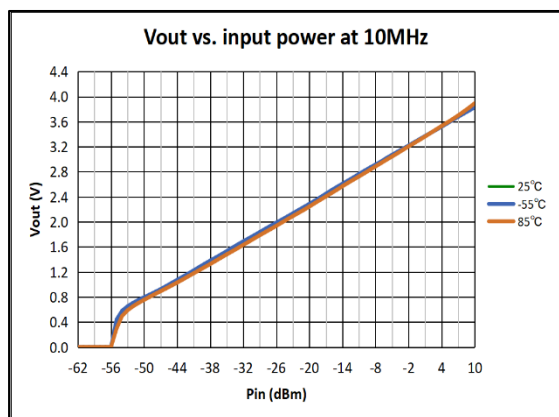
图 1 10MHz 全温检波曲线
