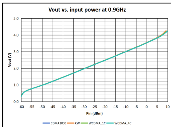
图 21 900MHz 调制信号检波曲线
