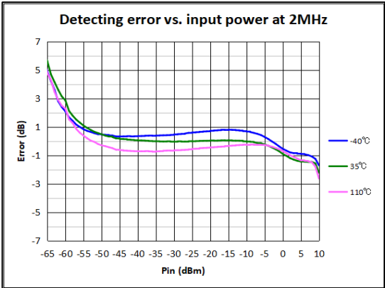
图 2 2MHz 全温检波对数误差
