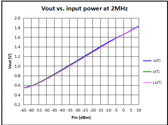
图 1 2MHz 全温检波曲线
