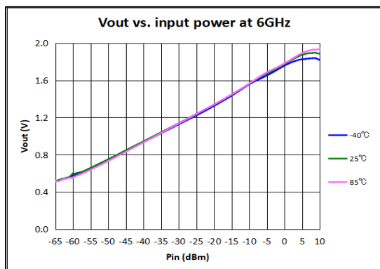
图 11 6000MHz 全温检波曲线
