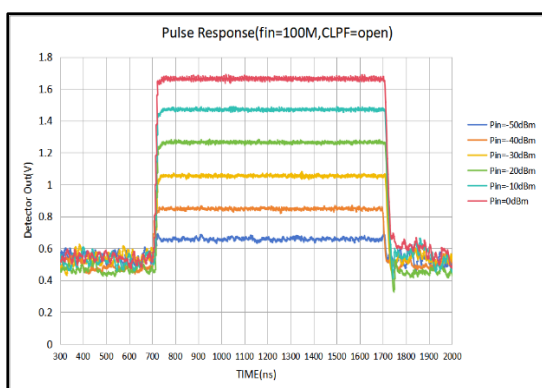
图 13 100MHz 输出瞬态响应, CLPF=Open
