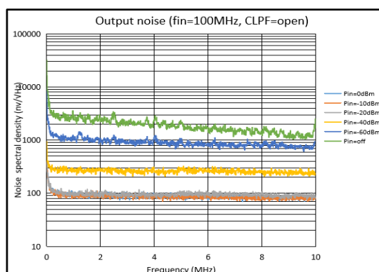
图 14 100MHz 输出噪声, CLPF=Open
