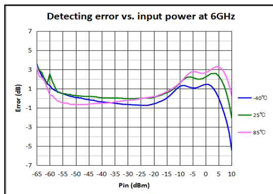
图 12 6000MHz 全温检波对数误差
